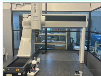
CNC三次元測定機 ミットヨ | CRISTAPEX9106 | 2016年 | 宮城県
