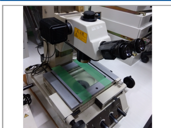
測定顕微鏡 ミットヨ | 176-842 | 不明年 | 埼玉県
